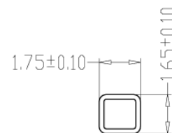
SEC:D-D
